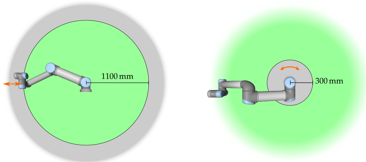
Figur 2.1: Spesielle områder til arbeidsplassen bør få oppmerksomhet angående klemmefare, som følge av robotarmens fysiske egenskaper. Et område defineres for radiale bevegelser, når håndleddet er på en avstand på minst 1100 mm fra basen til roboten. Det andre området er innen 300 mm fra basen til roboten, når den beveger seg i den tangentielle retningen.
