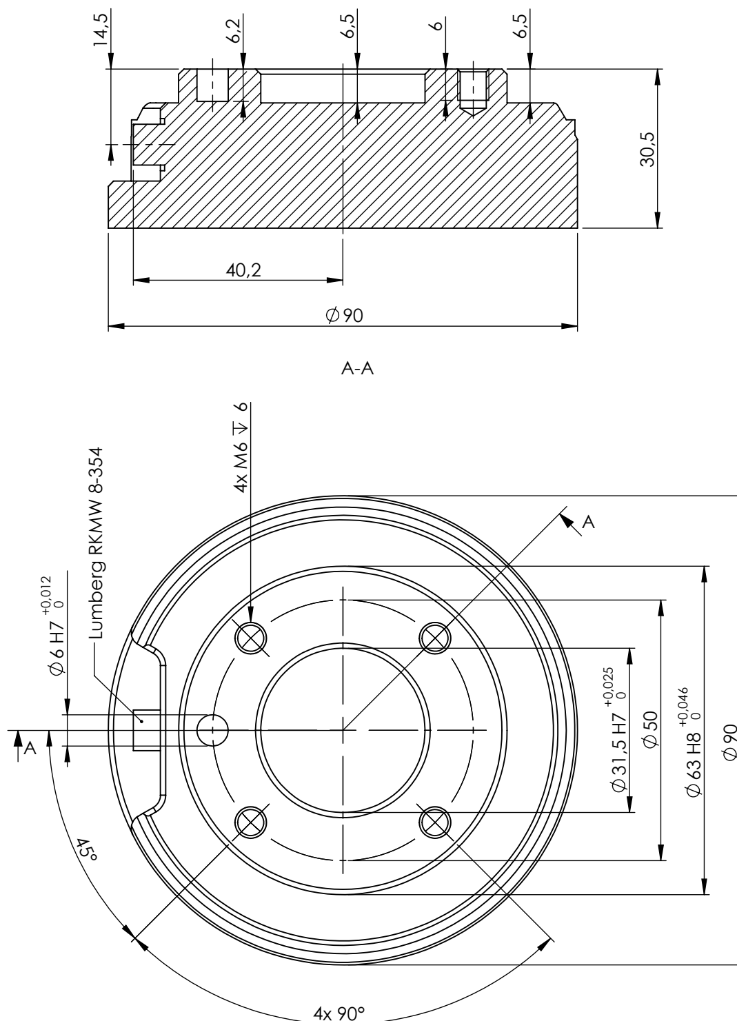
Figur 4.2: Verktøyutgangsf lens, ISO 9409-1-50-4-M6. Dette er hvor verktøyet monteres på tuppen av roboten. Alle mål er i mm.
