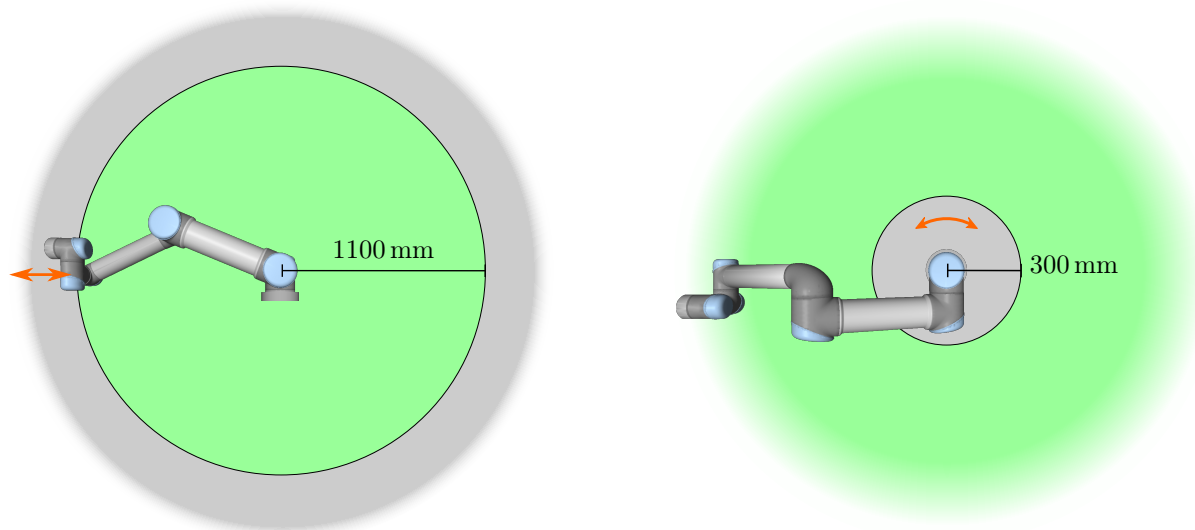
Рис. 2.1: Определенным рабочим зонам должно быть уделено особое внимание в части угроз защемления, связанных с физическими свойствами манипулятора робота. Одна зона отведена под радиальные перемещения, при которых запястье 1 сочленения находится на расстоянии менее 1100 мм от основания робота. Другая зона находится в пределах 300 мм от основания робота в случае перемещения по касательной.
