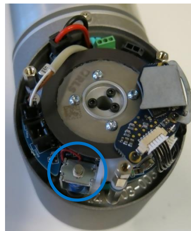
手首ジョイントのブレーキ
