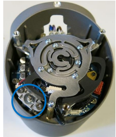
손목 조인트의 브레이크
