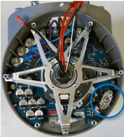
베이스 브레이크 및 숄더 조인트
