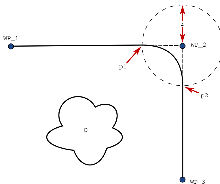
43.1: Overgang over ( WP\_2 ) med radius ( r ), første overgangsposition ved p1 og endelige overgangsposition ved p2 . ( O ) er en forhindring.
