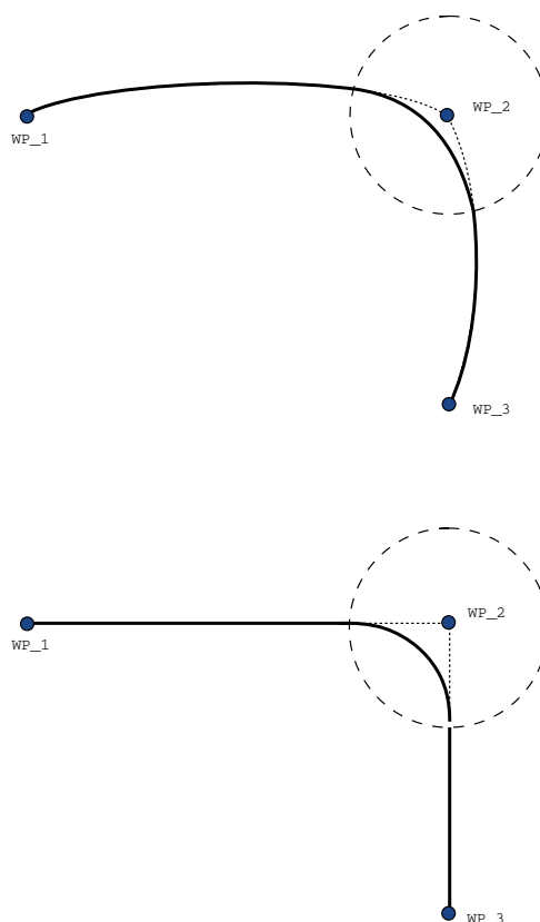
44.1: Fælles rum ( MoveJ ) vs. kartesisk rum ( MoveL ) bevægelse og blanding.
