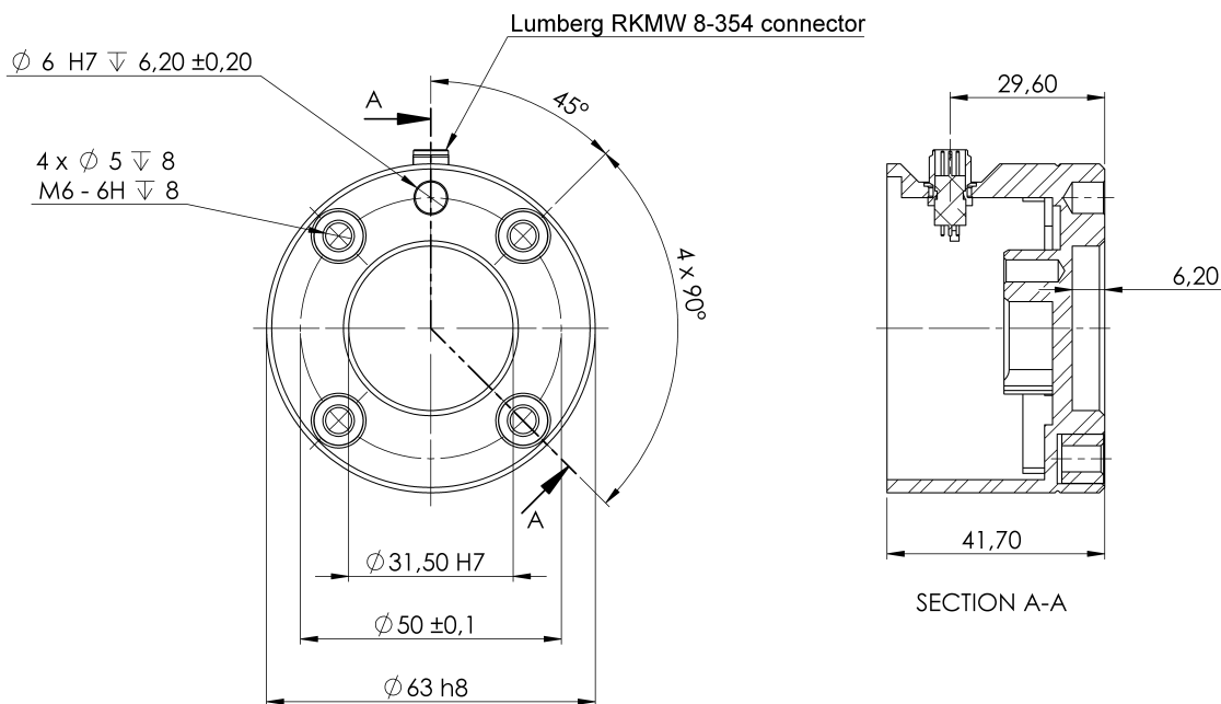
3.1: Værktøjsflangens mål og hulmønster. Alle mål er i mm.
