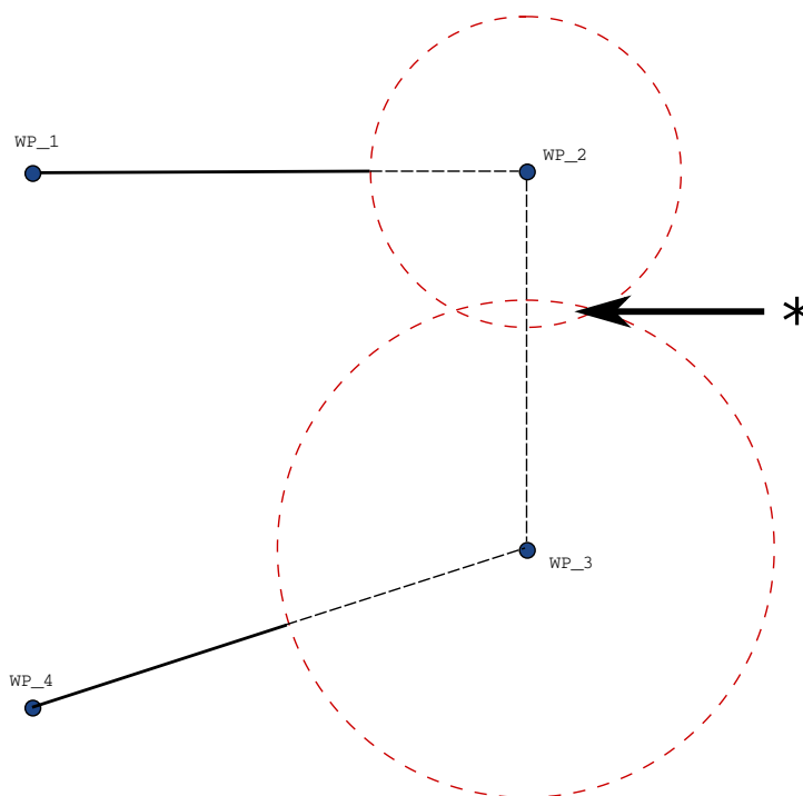
43.2: Overlapning af blandingsradius er ikke tilladt (*).
