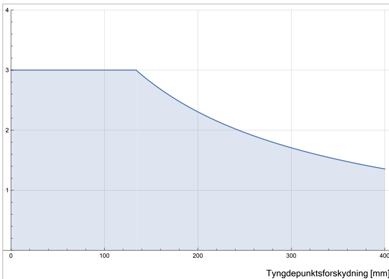
3.2: Forholdet mellem den nominelle nyttelast og tyngdepunktet forskydes.
