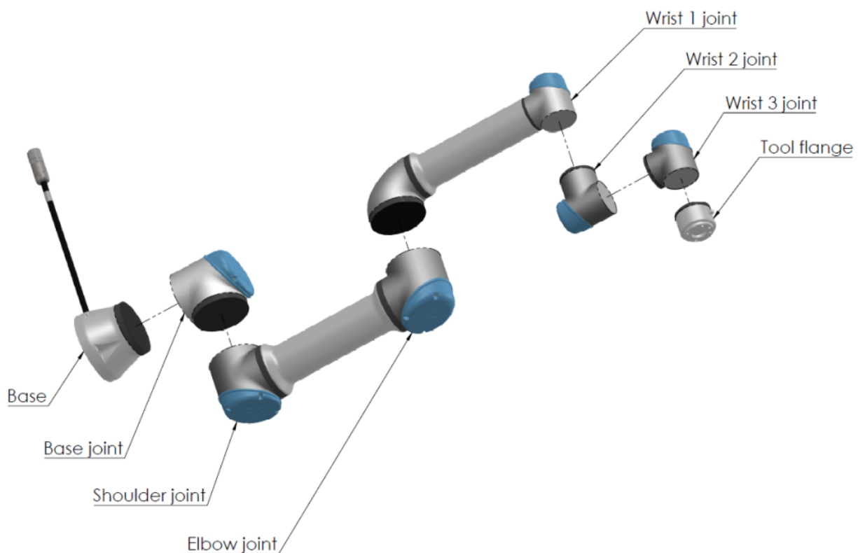
1.1: Die Gelenke, die Basis und der Werkzeugflansch am Roboterarm.
