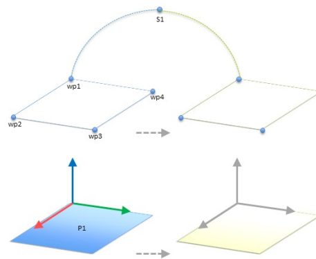
65.1: Einfaches Programm mit vier Wegpunkten relativ zu einer Funktionsebene manuell aktualisiert, indem die Funktion geändert wird
