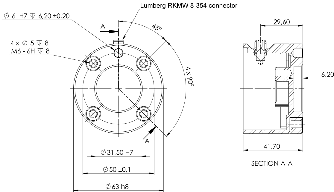
3.1: Abmessungen und ein Lochbild des Werkzeugflanschs. Alle Maße sind in mm.
