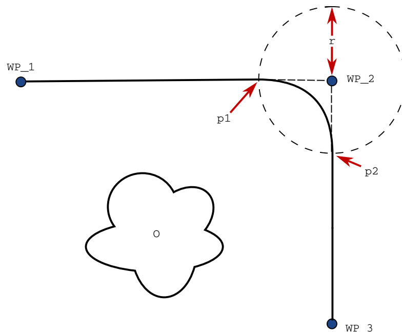
42.1: Überblendung über ( WP\_2 ) mit Radius ( r ), Anfangsposition der Überblendung bei p_1 und Endposition der Überblendung bei p_2 . (O) ist ein Hindernis.
