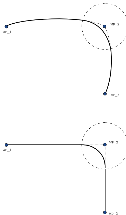
43.1: Gelenkraum ( MoveJ ) vs. kartesischer Raum ( MoveL ) Bewegung und Mischung.
