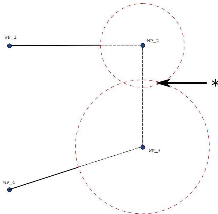
42.2: Überlappung des Mischradius nicht zulässig (*).
