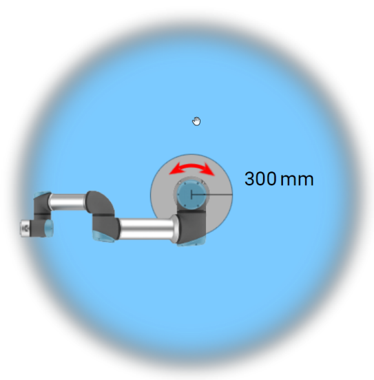
1.2: 由于机器人手臂的物理特性，某些工作区需要注意夹伤危险。其中一个区域(左)是定义的径向运动区域，即手腕 1 关节与机器人基座至少相距 800 mm 的区域。另一个区域(右)是在机器人基座 300 mm 范围内的区域(机器人按正切方向移动时)。
