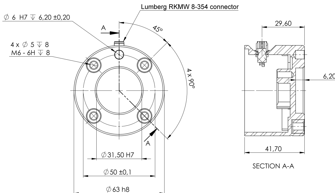
3.1: Værktøjsflangens mål og hulmønster. All measures are in mm.
