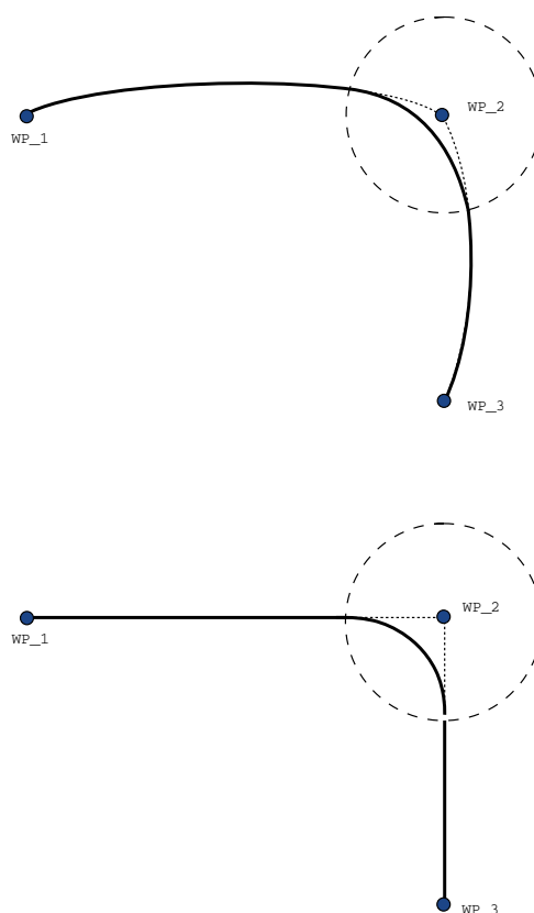
41.1: Fælles rum ( MoveJ ) vs. kartesisk rum ( MoveL ) bevægelse og blanding.
