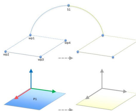
62.1: Enkelt program med fire waypoints i forhold til et funktionsplan manuelt opdateret ved at ændre funktionen
