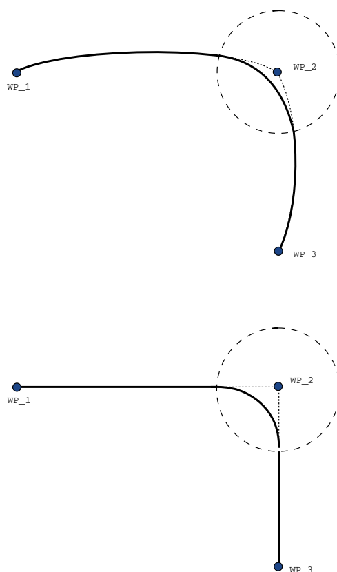
41.1: Spaziatura articolare ( MoveJ ) vs. spazio cartesiano ( MoveL ) movimento e sfumatura.
