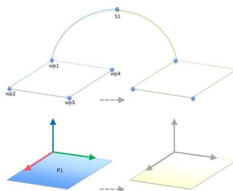
62.1: Programma semplice con quattro waypoint relativi ad un piano di feature aggiornato manualmente modificando la feature
