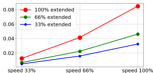
Distanza di arresto in metri per un carico utile massimo di 3 kg
