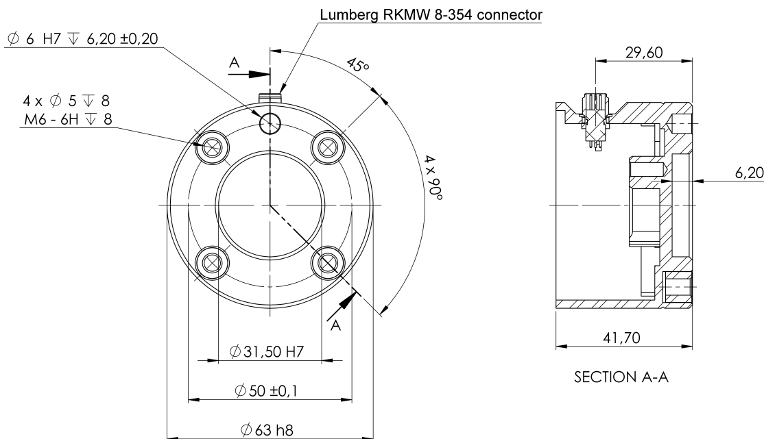
3.1: Dimensioni e schema dei fori della flangia dell'utensile. All measures are in mm.
