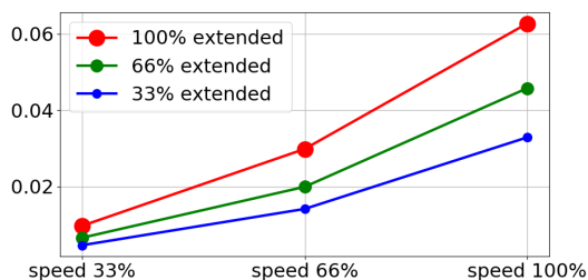
Distanza di arresto in metri per il 33% di 3kg
