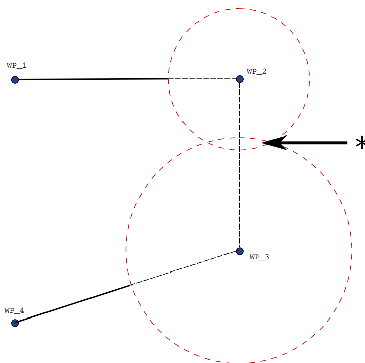
40.3: Sovrapposizione raggio miscela non consentita (*).
