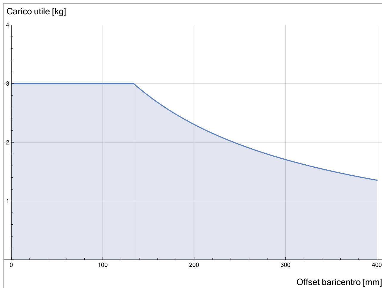
3.2: Rapporto fra il carico utile nominale e l'offset del centro di gravità.
