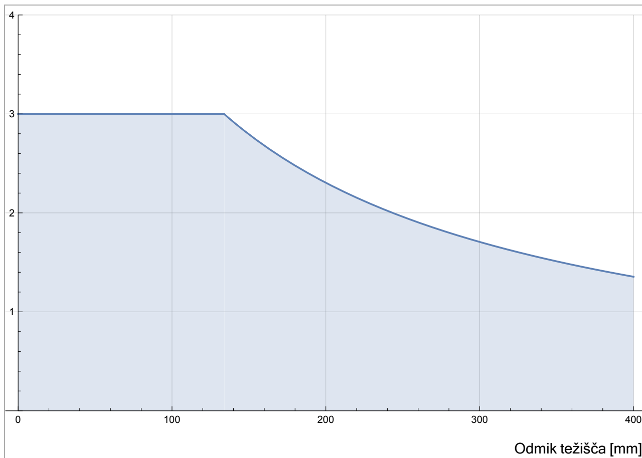
3.2: Razmerje med nazivno obremenitvijo in odmikom težišča.
