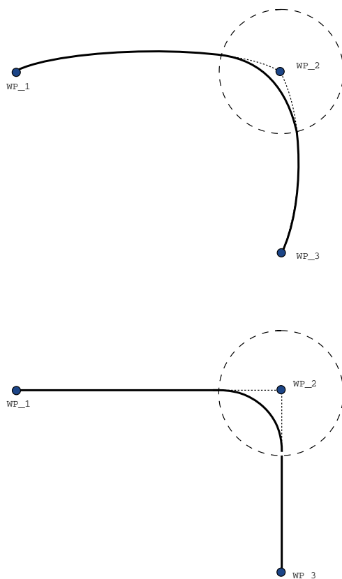
41.1: Gibanje in mešanje skupnega prostora ( MoveJ ) v primerjavi s kartezičnim prostorom ( MoveL ).
