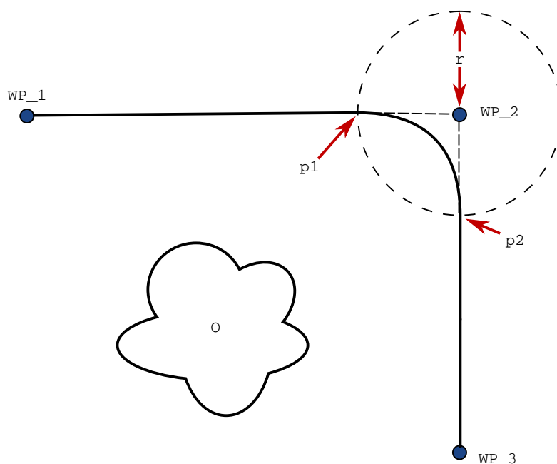
40.2: Spoj preko ( WP\_2 ) z radijem ( r ), začetni položaj spoja pri p1 in končni položaj spoja pri p2 . ( O ) je ovira.
