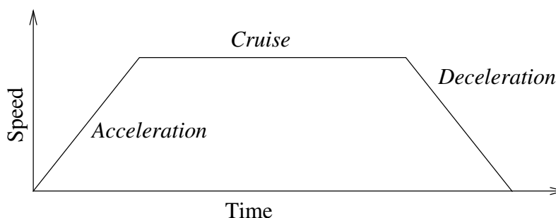
29.1: Hastighedsprofil for en bevægelse. Kurven er opdelt i tre segmenter: acceleration, cruise og deceleration. Niveauet for cruise-fasen bestemmes ved indstilling af hastigheden for bevægelsen, mens stejlheden i faserne med acceleration og deceleration bestemmes af accelerationsparameteret.
