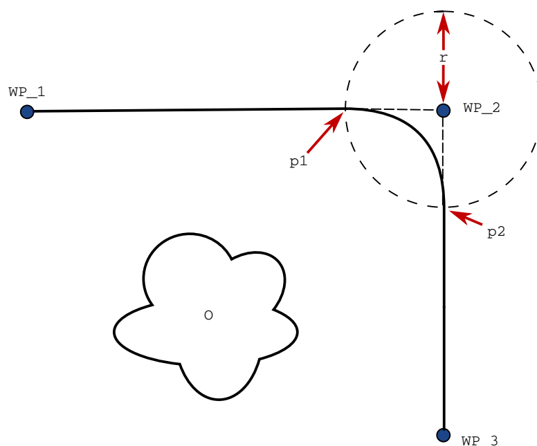
31.2: Overgang over ( WP\_2 ) med radius ( r ), første overgangsposition ved p1 og endelige overgangsposition ved p2 . ( O ) er en forhindring.
