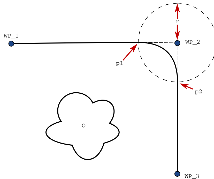
31.2: Überblendung über ( WP\_2 ) mit Radius ( r ), Anfangsposition der Überblendung bei p_1 und Endposition der Überblendung bei p_2 . ( O ) ist ein Hindernis.
