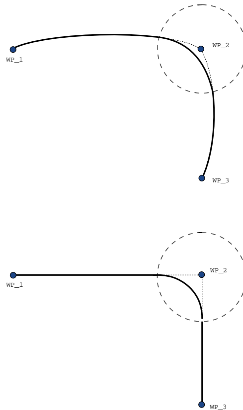
32.1: Gelenkraum ( MoveJ ) vs. kartesischer Raum ( MoveL ) Bewegung und Mischung.
