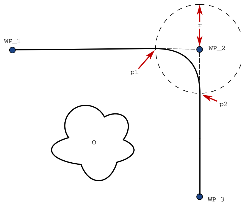
31.2: Transizione lungo ( WP\_2 ) con raggio ( r ), posizione di transizione iniziale in p1 e posizione di transizione finale in p2 . ( O ) è un ostacolo.
