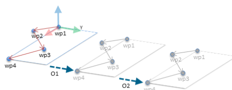
53.3: Applicazione di un offset alla caratteristica del piano
