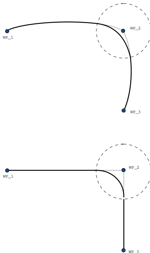
32.1: Spaziatura articolare ( MoveJ ) vs. spazio cartesiano ( MoveL ) movimento e sfumatura.
