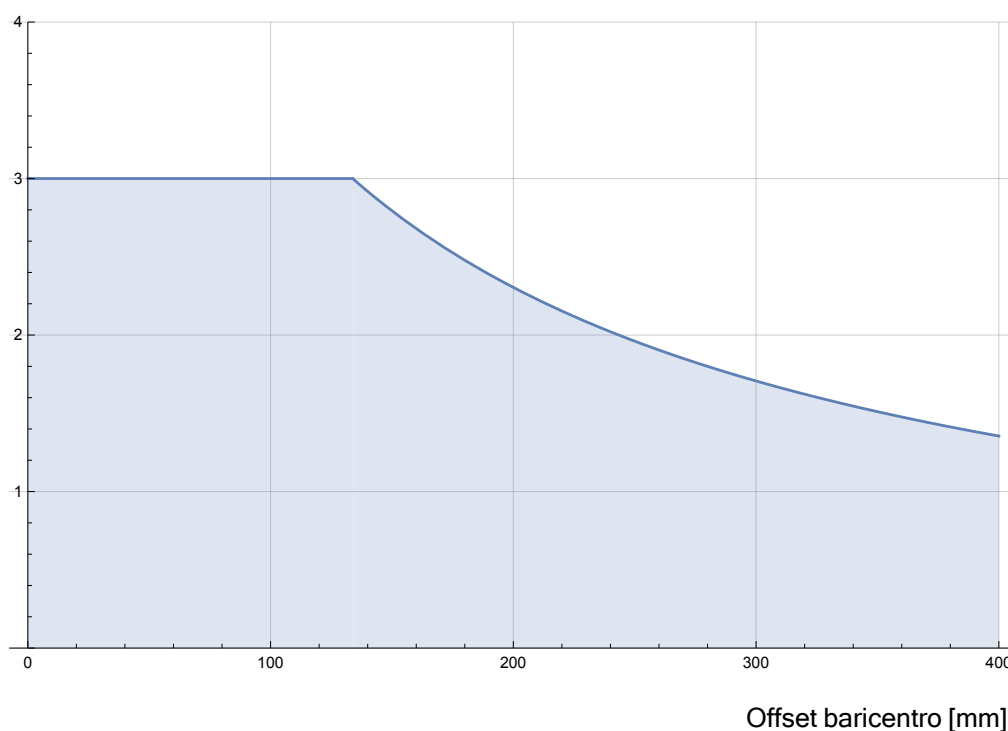
1.3: Rapporto fra il carico utile nominale e l'offset del centro di gravità.
