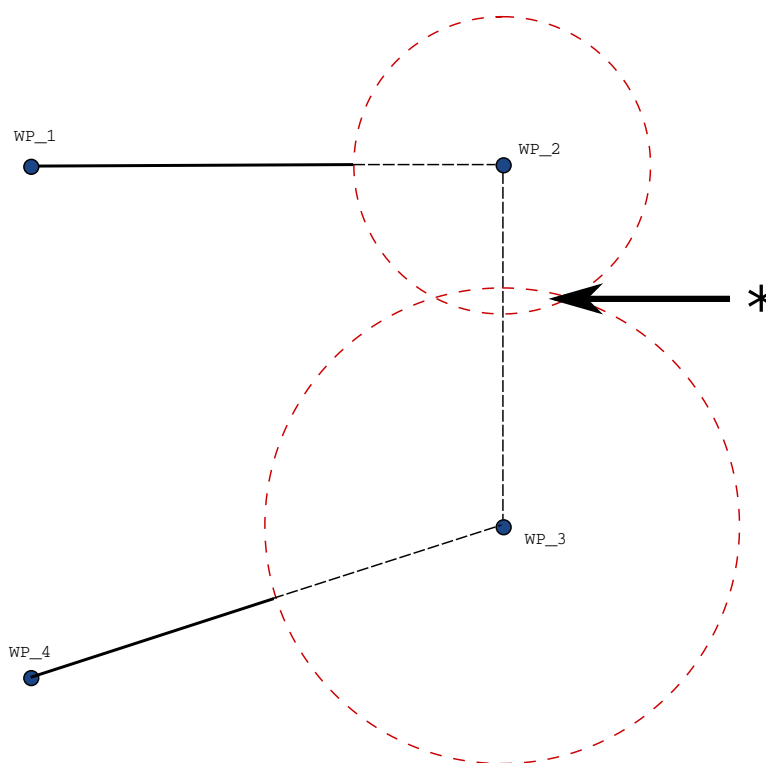
31.3: Sovrapposizione raggio miscela non consentita (*).
