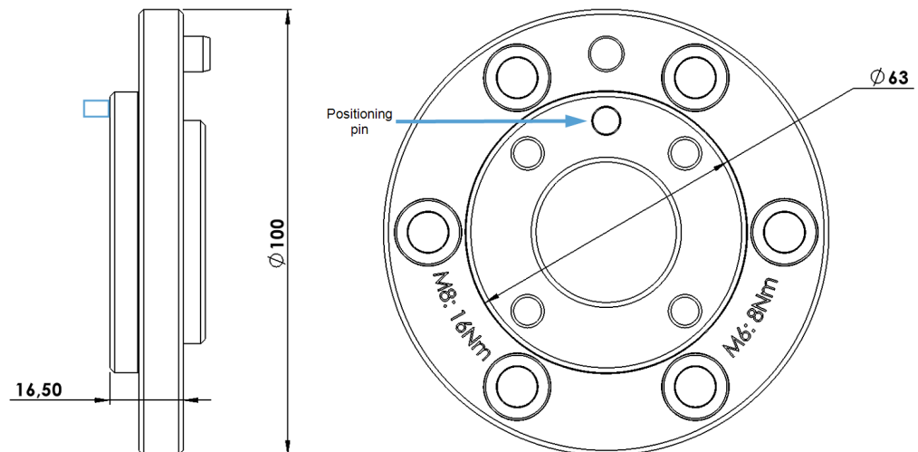
Abmessungen und Schraubenanzugsmomente des Werkzeugflanschadapters.
