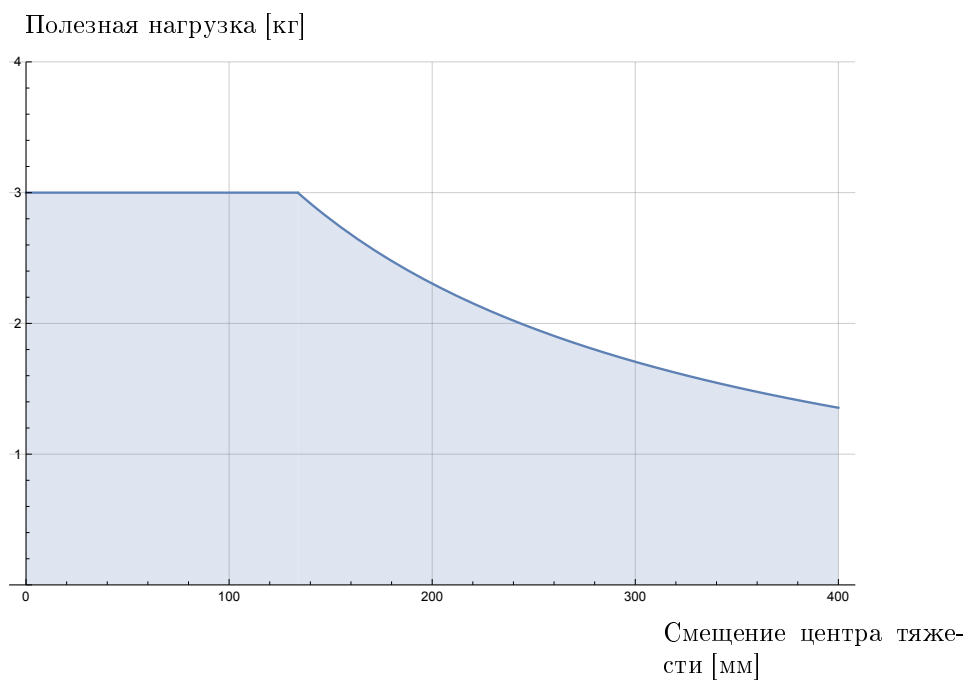
Рис. 4.3: Соотношение между максимально допустимой полезной нагрузкой и смещением центра тяжести.
