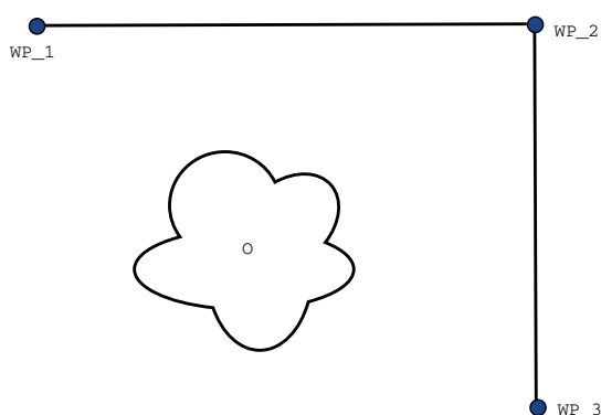
Рис. 14.2: WP_1: начальное положение, WP_2: промежуточная точка, WP_3: положение захвата, O: препятствие.
