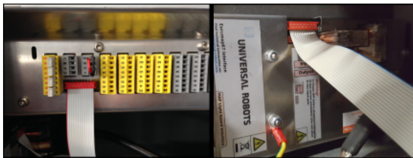
Рис. 19.1: Подключение шлейфа
