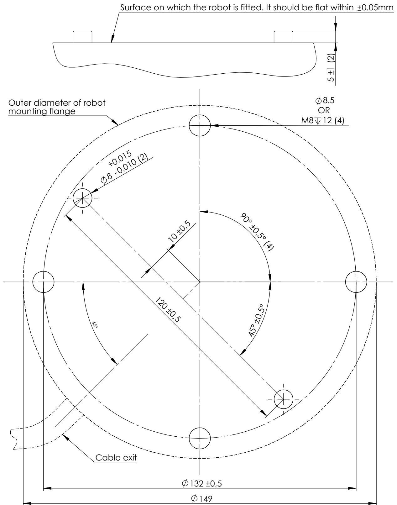
Рис. 4.1: Отверстия для монтажа робота. Используются четыре M8 болта. Все измерения приведены в мм.
