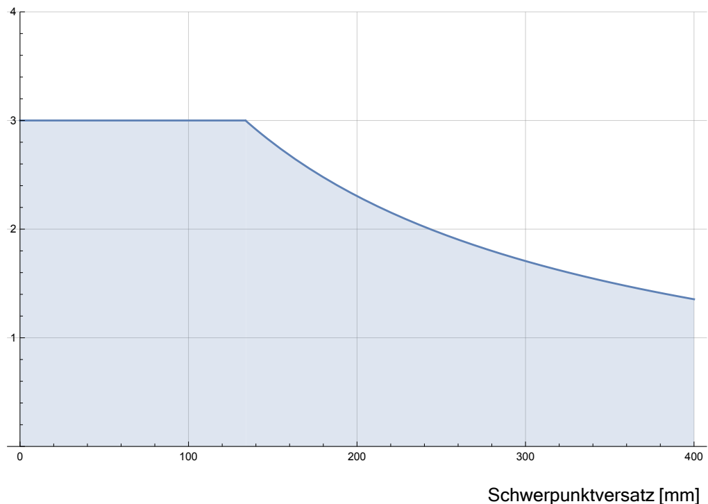
1.3: Beziehung zwischen der Nennnutzlast und der Schwerpunktverschiebung.
