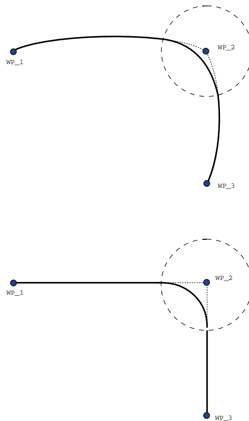
11.1: Gelenkraum ( MoveJ ) vs. kartesischer Raum ( MoveL ) Bewegung und Mischung.
