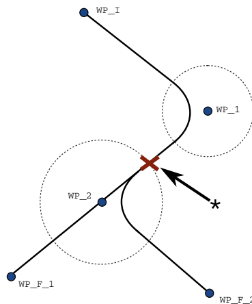
11.2: WP_I ist der anfängliche Wegpunkt und es gibt zwei mögliche endgültige Wegpunkte WP_F_1 und WP_F_2, abhängig von einem bedingten Ausdruck. Die Bedingung if wird ausgewertet, sobald der Roboterarm die zweite Überblendung (*) erreicht.
