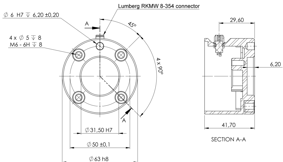
1.2: 툴의 치수 및 구멍 패턴. 모든 측정 단위는 mm 입니다.
