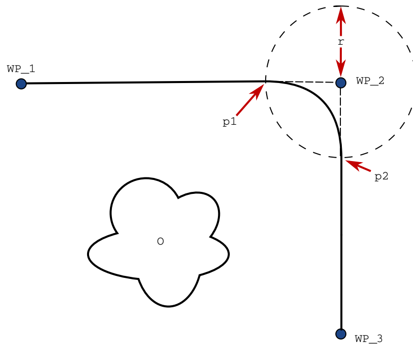
11.2: ( r ) 반지름을 ( WP\_2 )에 적용하여 혼합하고, 최초 위치는 p1 , 최종 위치는 p2 입니다. ( O )는 장애물입니다.
