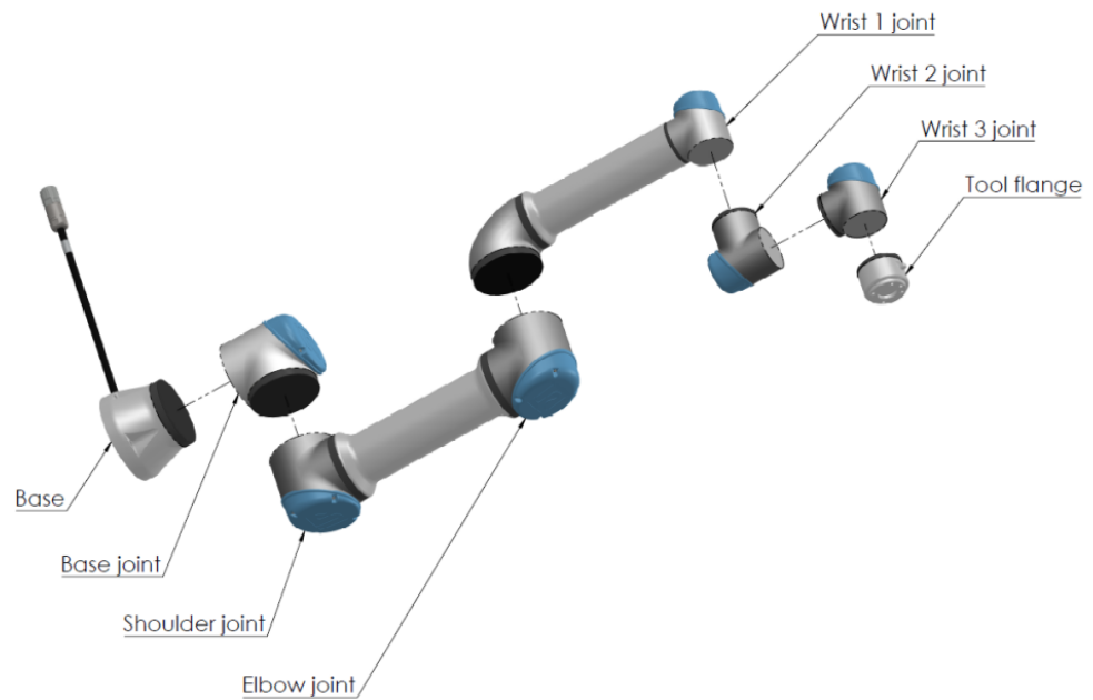
1.1: 로봇 암의 조인트, 베이스 및 툴 플랜지.
