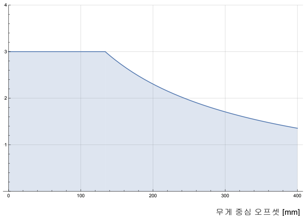
1.3: 정격 페이로드와 무게중심 오프셋 간의 관계.
