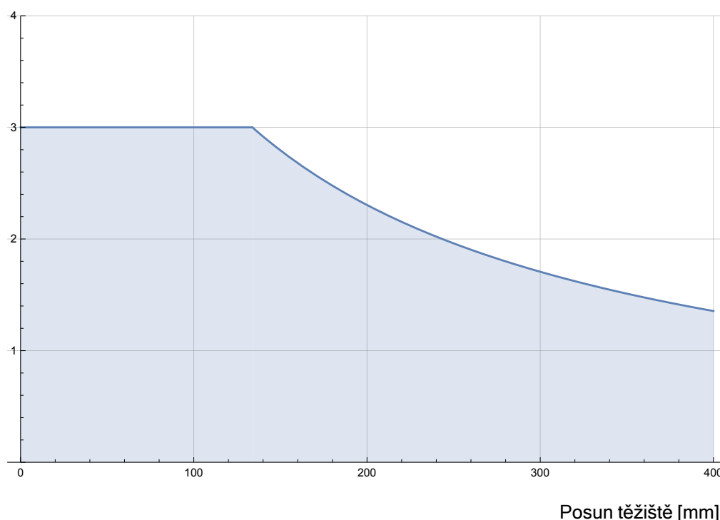
1.3: Vztah mezi jmenovitým užitečným zatížením a posunem těžiště.
