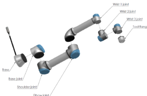
1.1: Hlavní součásti robotického ramene.
