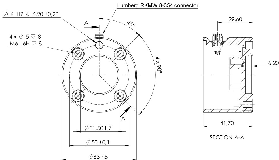
1.2: Rozměry a rozmístění otvorů nástroje. Všechny míry jsou uvedeny v milimetrech.
