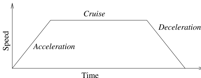
11.1: Profilo di velocità di un movimento. La curva è suddivisa in tre segmenti: accelerazione, crociera e decelerazione. Il livello della fase di crociera deriva dall'impostazione della velocità del movimento, mentre la ripidità delle fasi di accelerazione e decelerazione derivano dal parametro di accelerazione.
