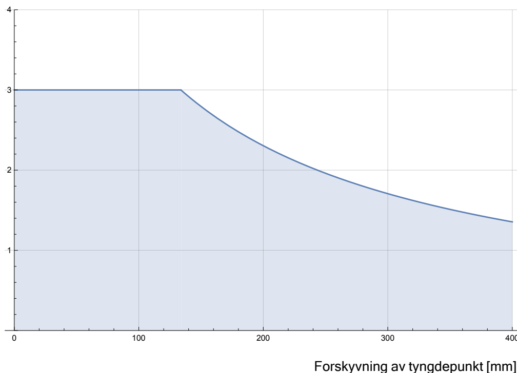
1.3: Forholdet mellom rangert nyttelast og forskyvningen av tyngdepunktet.
