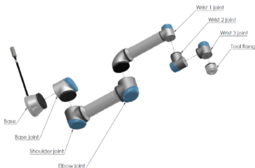
1.1: Robotarmens hovedkomponenter.
