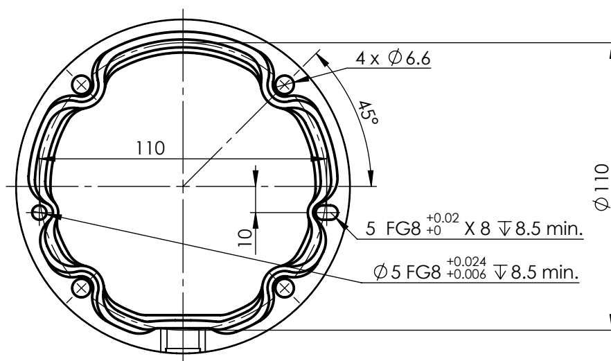
Dimensões e padrão de orifícios para a montagem do robot.
