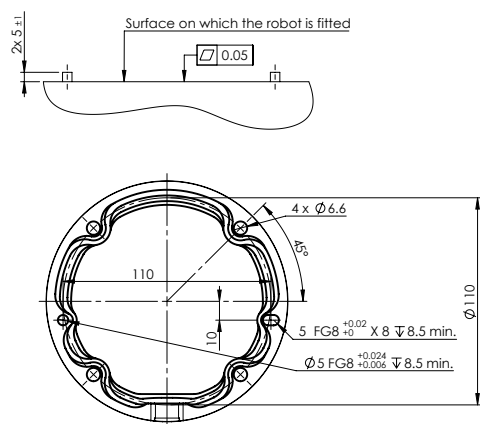
Mere in vzorec lukenj za pritrditev robota.
