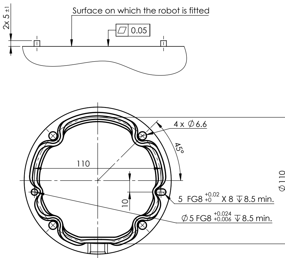
Mått och hålmönster för montering av roboten.
