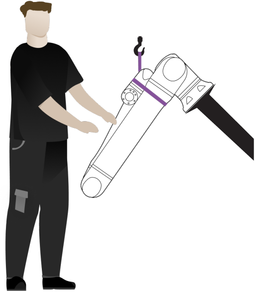
Açısal montaj ( \pm 45^\circ )
