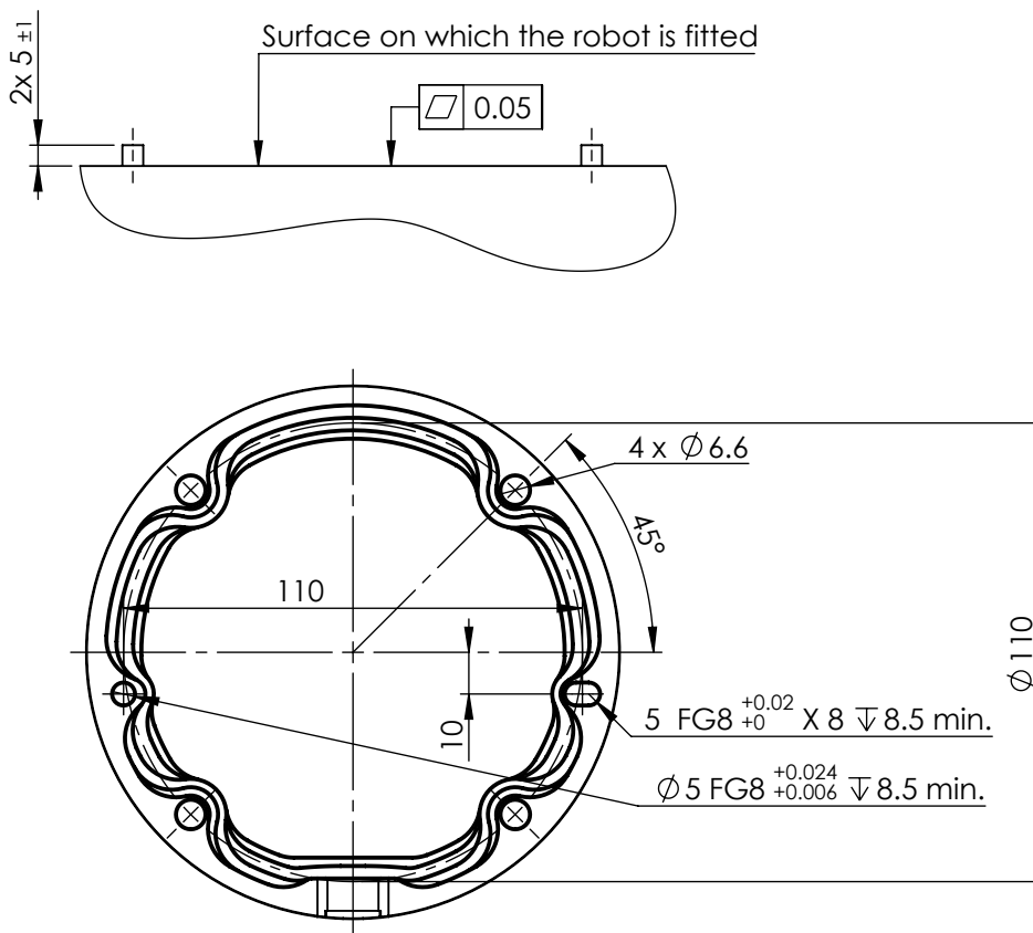
Méreték és furatkép a robot felszereléséhez.
