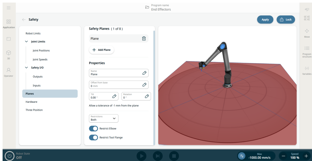
Ábra 1.4 : PolyScope X képernyő megjelenített biztonsági síkokkal.
