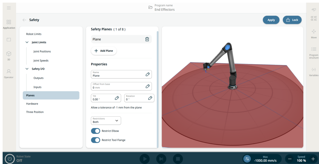
Rysunek 1.4: Ekran PolyScope X wyświetlający płaszczyzny bezpieczeństwa.
