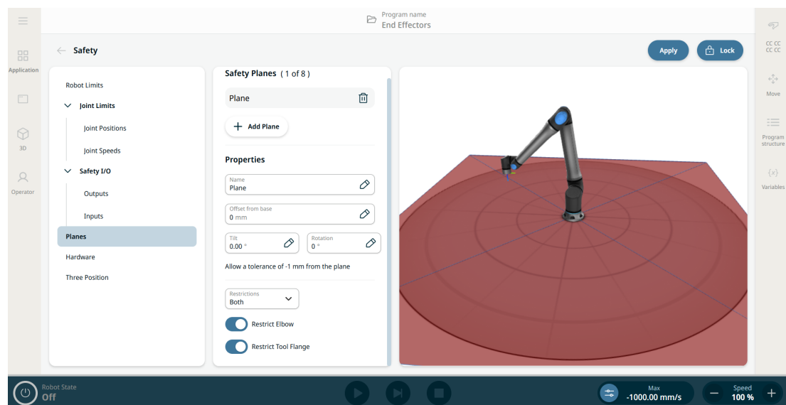
図 1.4: 安全平面を表示する PolyScope X 画面。
