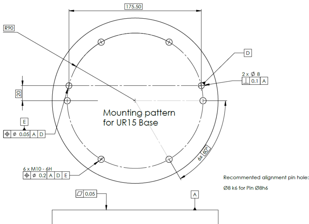
Dimensjoner og hullmønster for montering av roboten.
