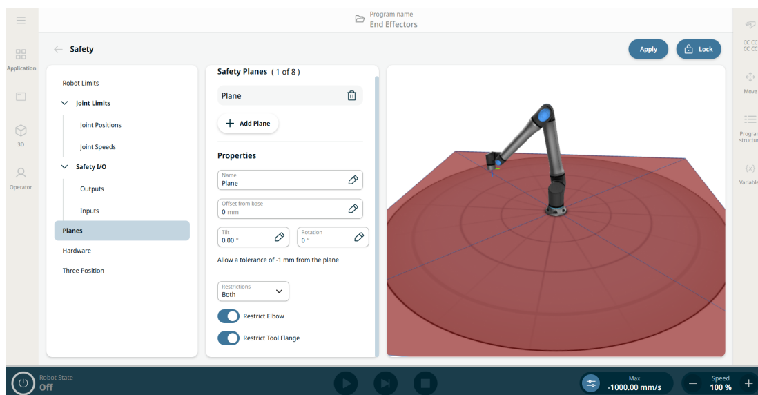
图 1.4: 显示了安全平面的 PolyScope X 屏幕。
