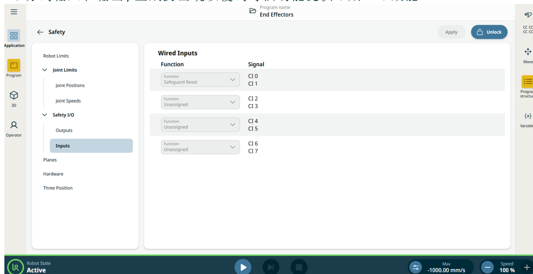
圖 1.3: 顯示輸入訊號的 PolyScope X 螢幕。
