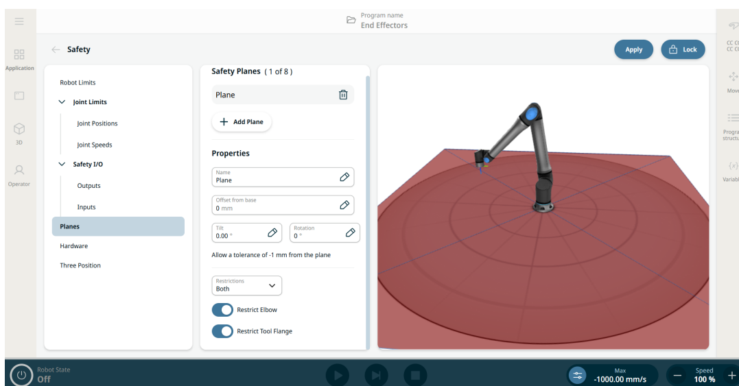
Číslo 1.4: Obrazovka PolyScope X zobrazující bezpečnostní roviny.
