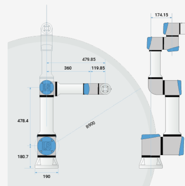
UR16e 尺寸和工作范围
