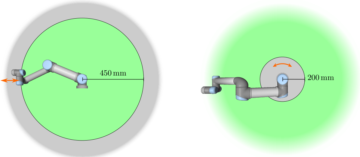
图 2.1: 鉴于机器人手臂的物理性质, 在工作区的某些区域应留意夹伤风险。其中一个区域是定义的径向运动区域, 即手腕 1 关节至少与机器人底座相距 450 mm 的区域。另一个区域是在机器人底座 200 mm 范围内的区域 (机器人按正切方向移动时)。
