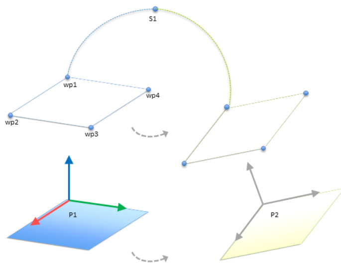
Abbildung 13.7: Umschalten von einer Ebenenfunktion zu einer anderen
