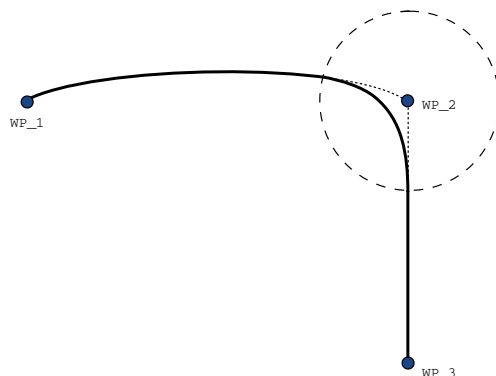
Obr. 14.7: Zatáčka z pohybu v spojenom priestore (PohybJ) do lineárneho pohybu nástroja (PohybL).
