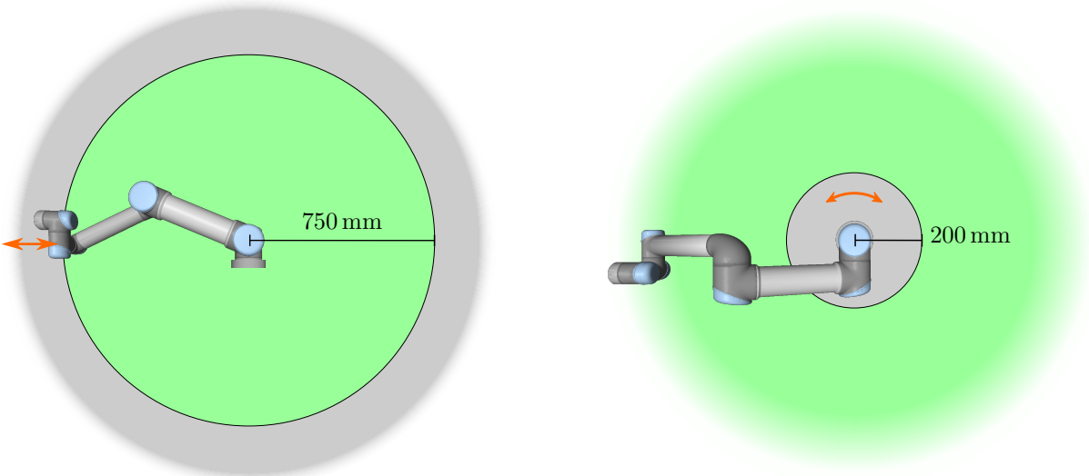
图 2.1: 鉴于机器人手臂的物理性质，在工作区的某些区域应留意夹伤风险。其中一个区域是定义的径向运动区域，即手腕 1 关节至少与机器人底座相距 750 mm 的区域。另一个区域是在机器人底座 200 mm 范围内的区域（机器人按正切方向移动时）。
