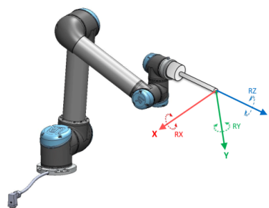
FIGURE 13.2 – Fonction de l'outil (point central de l'outil)
