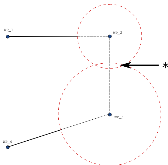
Figur 14.4: Overlapning af overgangsradius ikke tilladt (*).
