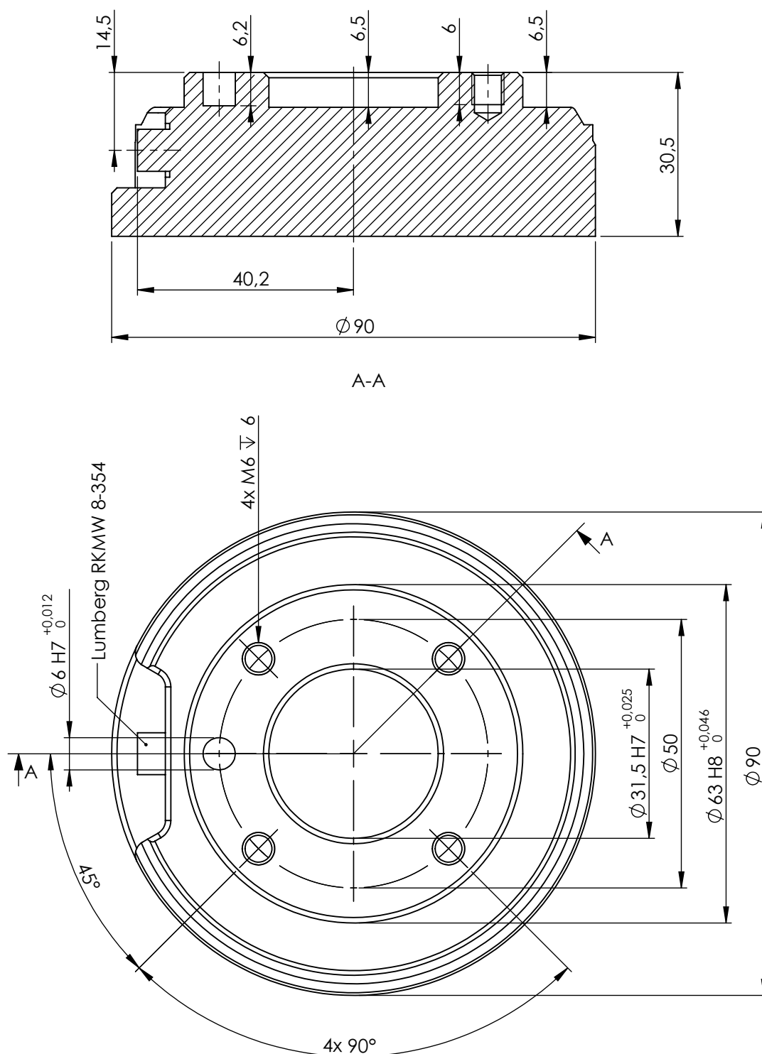
FIGURE 4.2 – La bride de sortie d’outil, ISO 9409-1-50-4-M6. À cet endroit, l’outil est monté sur l’extrémité du robot. Toutes les mesures sont en mm.
