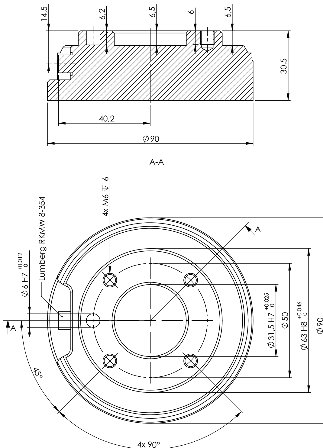
Рис. 4.2: Фланец для подсоединения инструмента, ISO 9409-1-50-4-M6. В этом месте инструмент прикрепляется к наконечнику робота. Все измерения приведены в мм.
