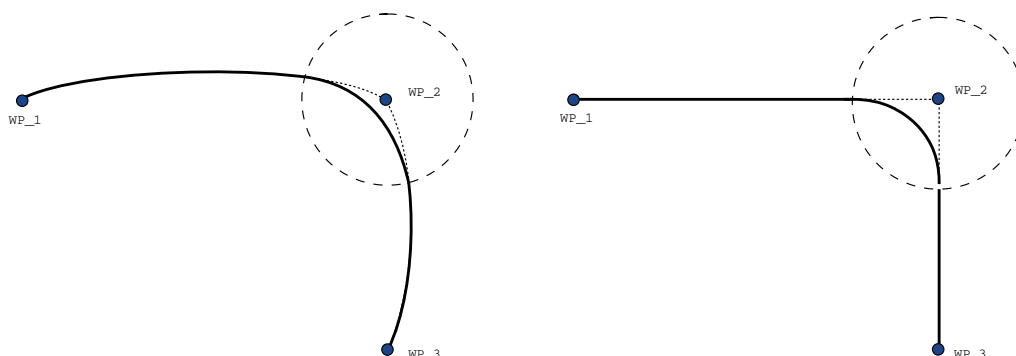
Obr. 14.6: Pohyb a zatăčenie v spojenom priestore (PohybJ) verzus karteziánskom priestore (PohybL).
