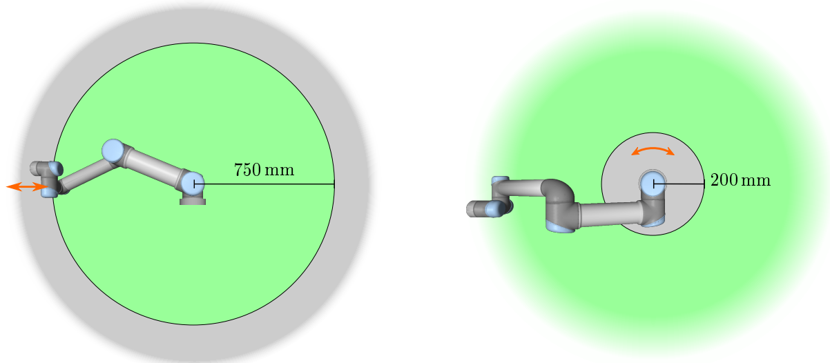
Figure 2.1: Определённым рабочим зонам должно быть уделено особое внимание в части угроз заземления, связанных с физическими свойствами манипулятора робота. Одна зона отведена под радиальные перемещения, при которых запястье 1 сочленения находится на расстоянии менее 750 мм от основания робота. Другая зона находится в пределах 200 мм от основания робота в случае перемещения по касательной.
