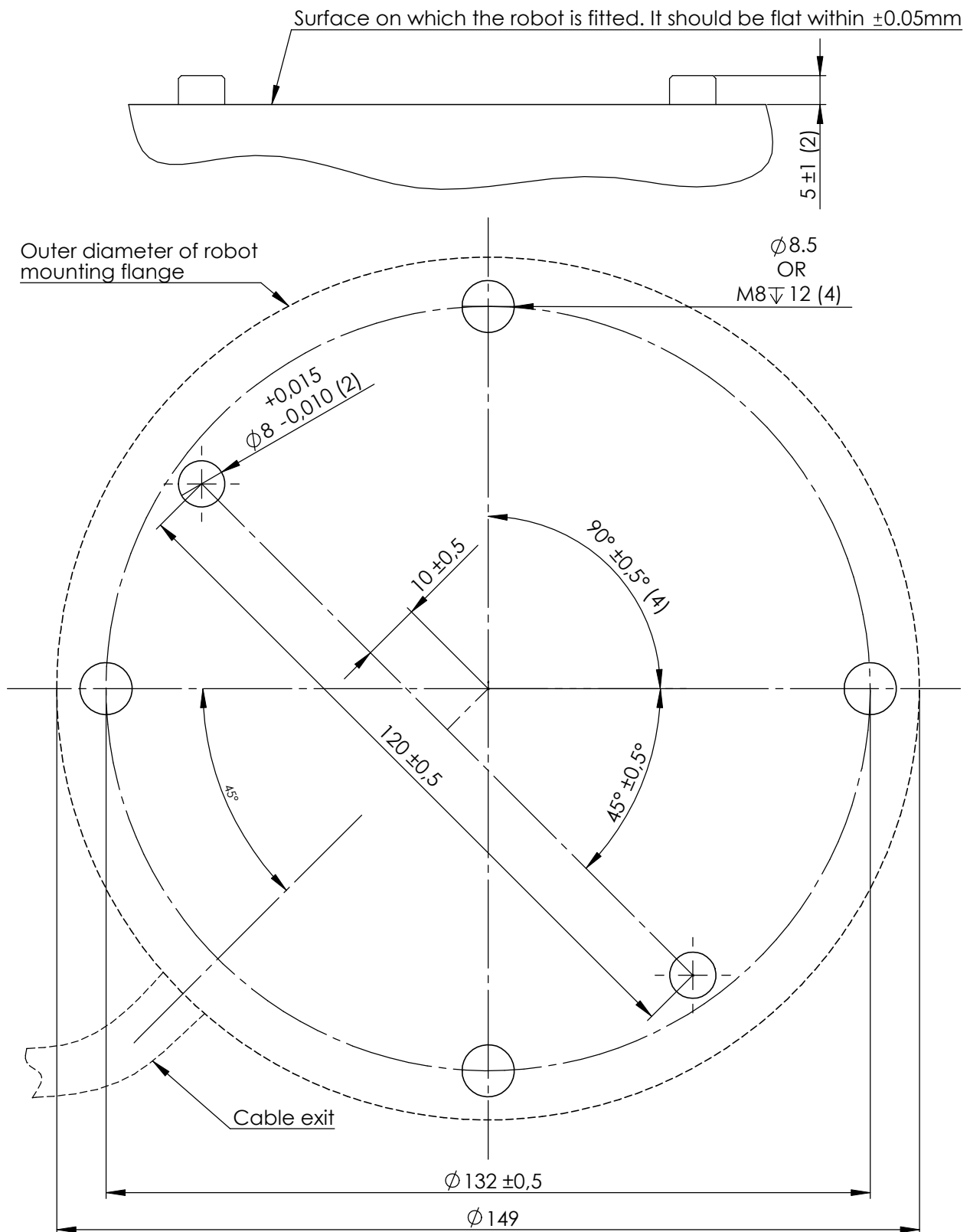
Figure 4.1: Отверстия для монтажа робота. Используются четыре M8 болта. Все измерения приведены в мм.
