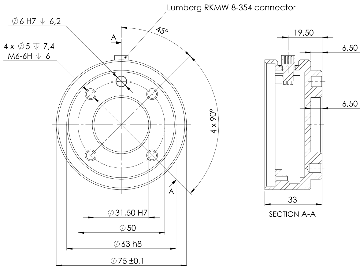
Figure 4.2: Фланец для подсоединения инструмента, ISO 9409-1-50-4-M6. В этом месте инструмент прикрепляется к наконечнику робота. Все измерения приведены в мм.
