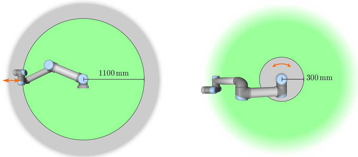
Figure 2.1: Определённым рабочим зонам должно быть уделено особое внимание в части угроз заземления, связанных с физическими свойствами манипулятора робота. Одна зона отведена под радиальные перемещения, при которых запястье 1 сочленения находится на расстоянии менее 1100 мм от основания робота. Другая зона находится в пределах 300 мм от основания робота в случае перемещения по касательной.
