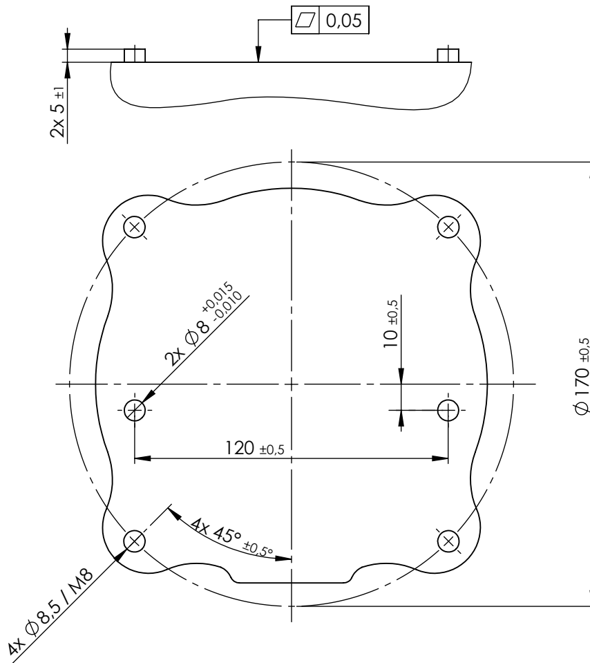
Figure 4.1: Отверстия для монтажа робота. Используются четыре M8 болта. Все измерения приведены в мм.
