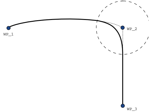
Şekil 14.7: Eklem alanındaki (Hareket Ettir J) bir hareketten doğrusal alet hareketine (Hareket Ettir L) harmanlama.
