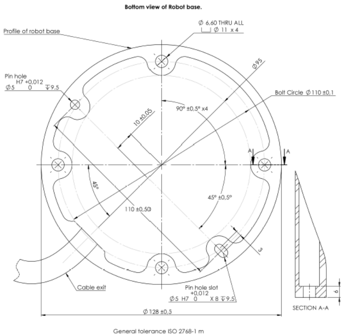
Figure 4.1: Отверстия для монтажа робота. Используются четыре M6 болта. Все измерения приведены в мм.
