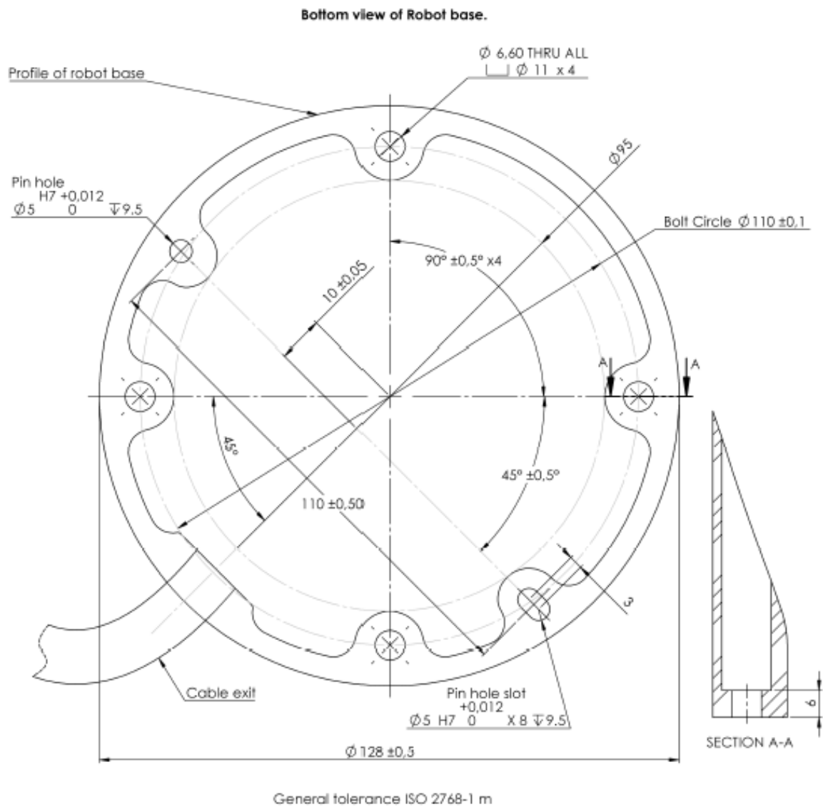
Obr. 4.1: Otvory na montáž robota. Použite štyri skrutky M6. Všetky merania sú v mm.
