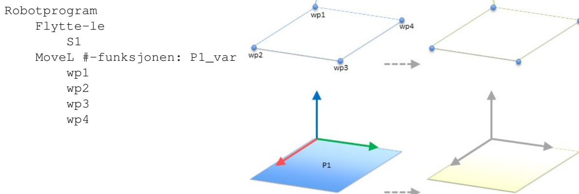
Figur 13.4: Enkelt program med fire veipunkter relativ til et funksjonsplan som blir manuelt oppdatert ved endring av funksjon
