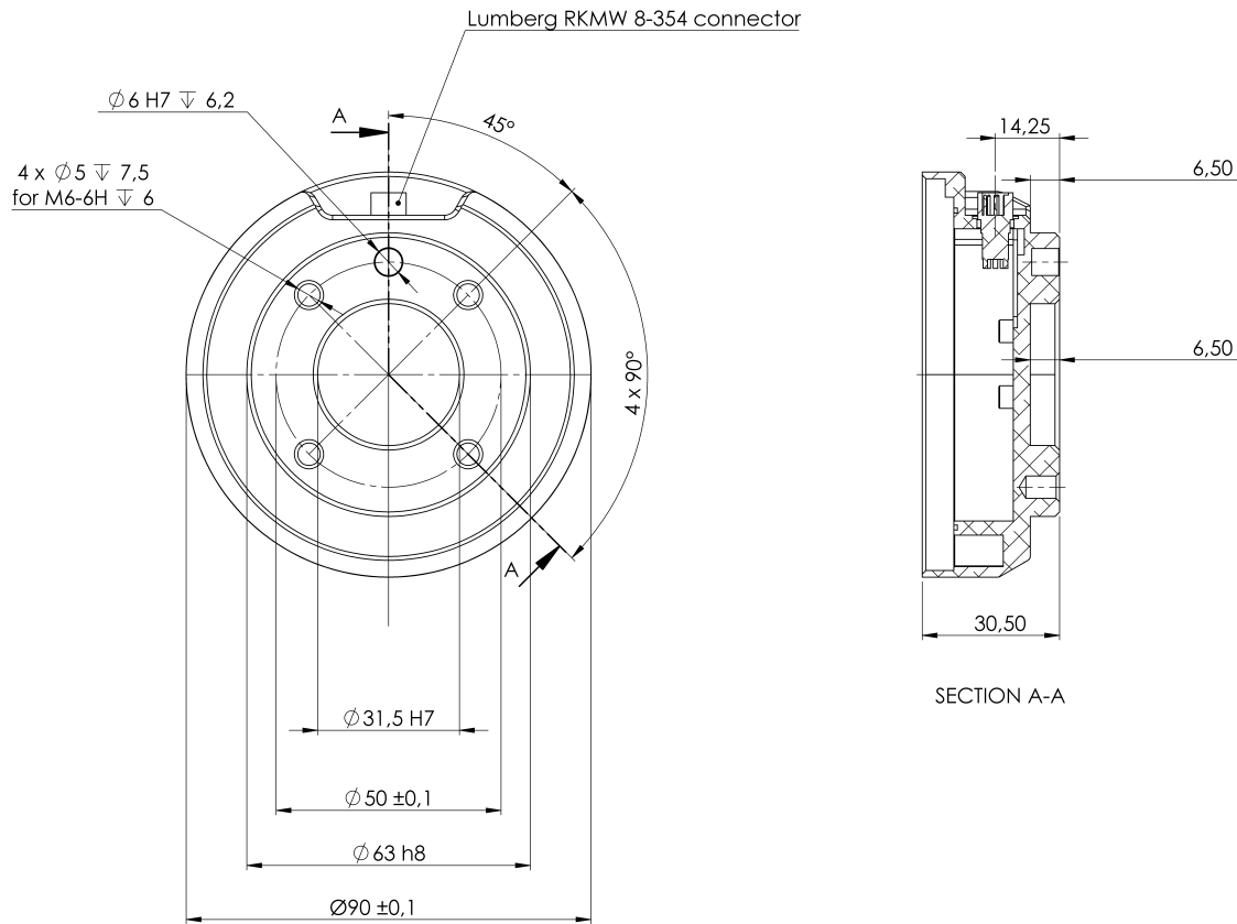
Figure 4.2: 툴출력플렌지, ISO 9409-1-50-4-M6. 여기가로봇끝에서툴을마운트하는위치이다. 모든측정단위는 mm 이다.
