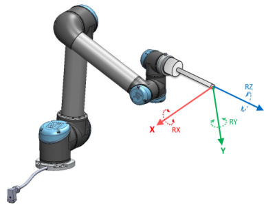
Figura 16.2: Funzione utensile (TCP)
